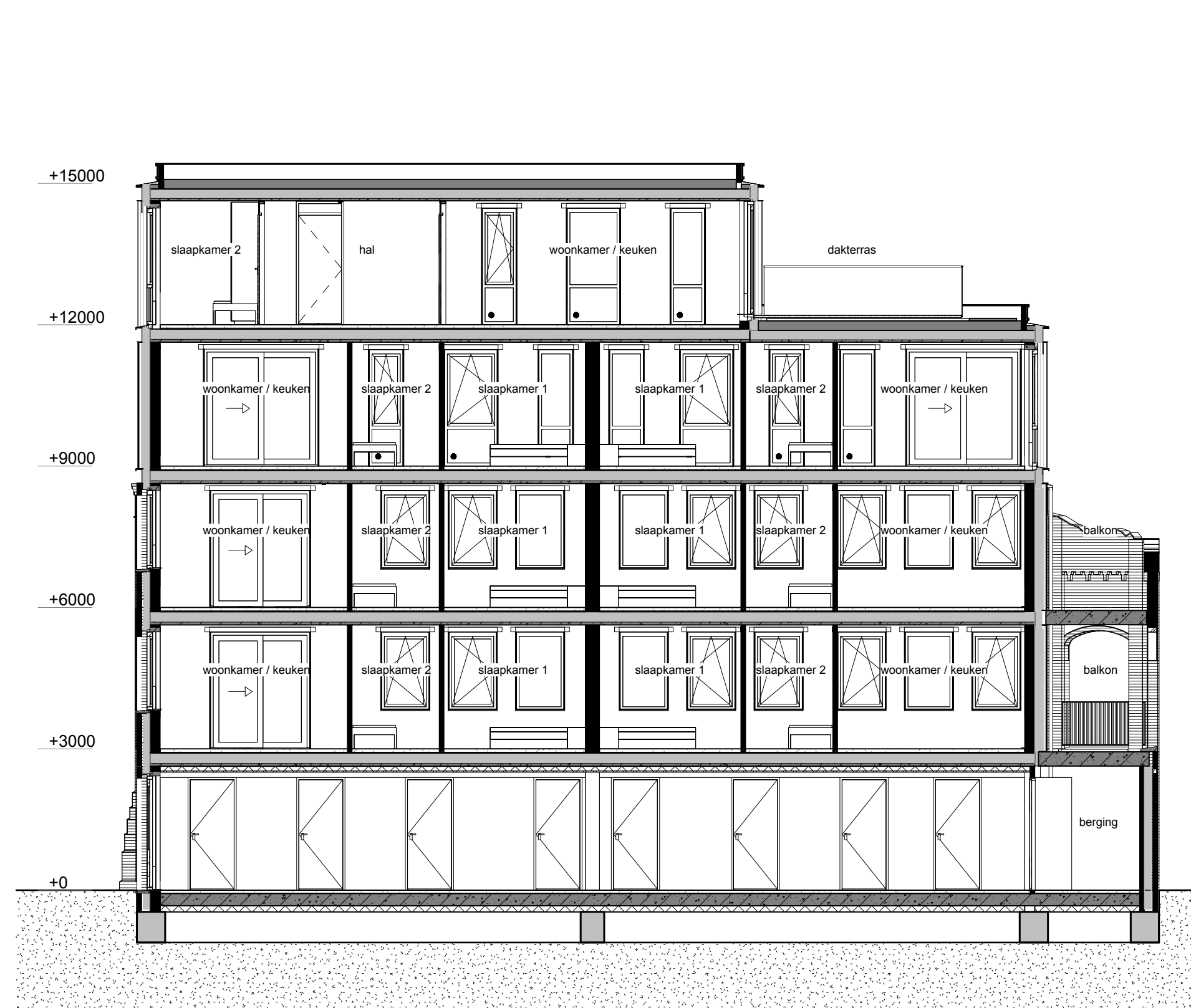
doorsnede A-A
