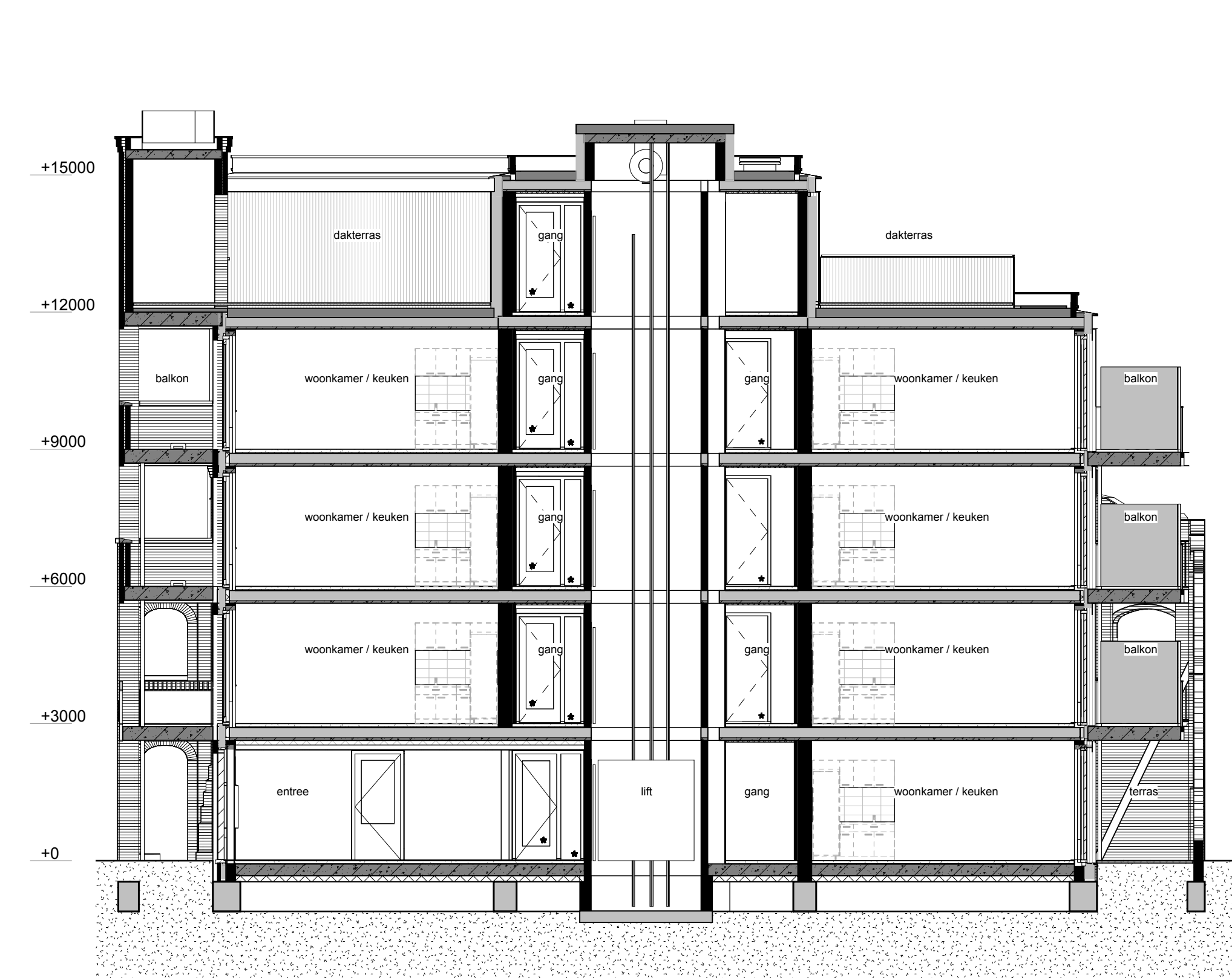
doorsnede B-B
