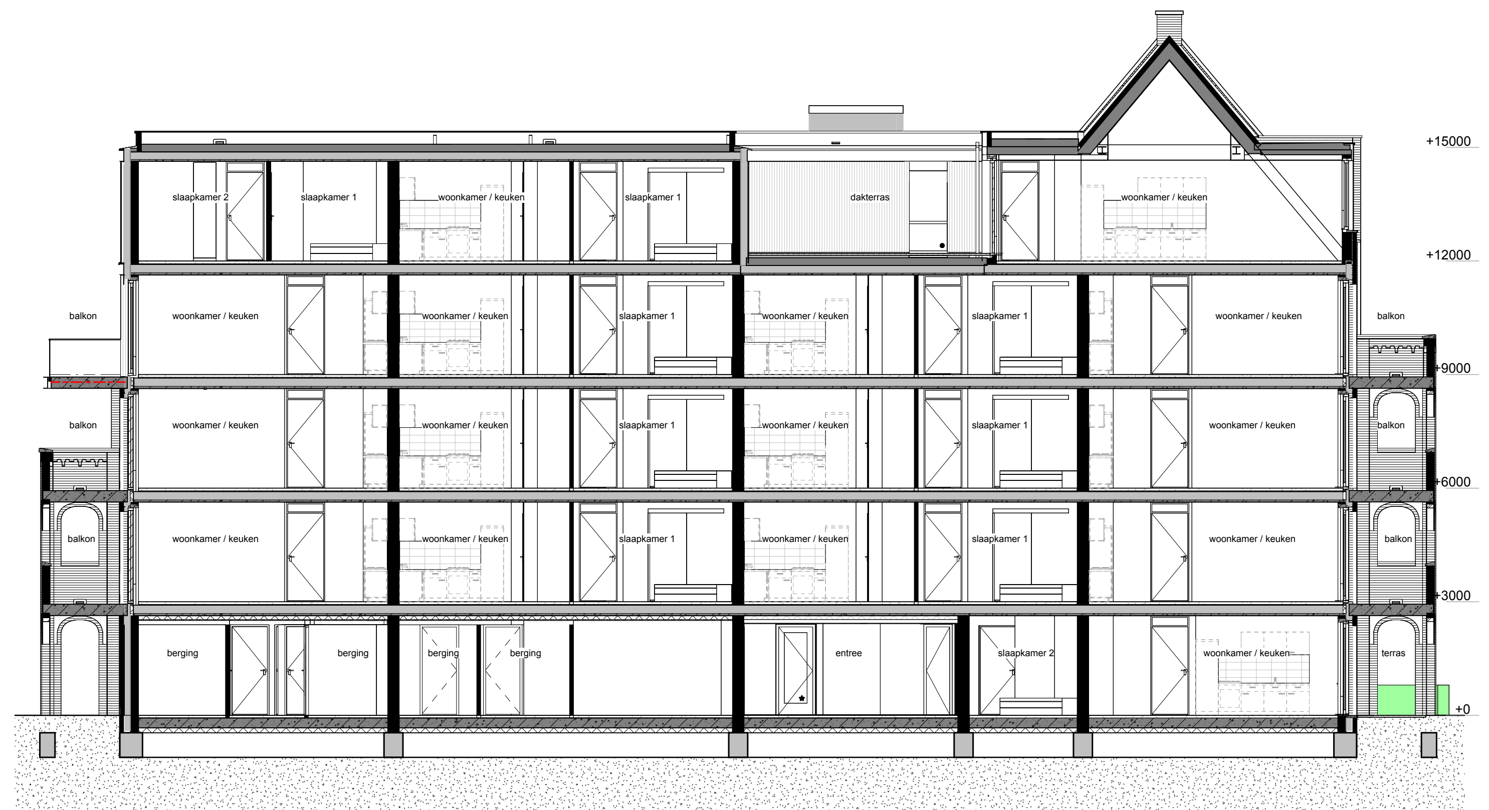
doorsnede C-C
